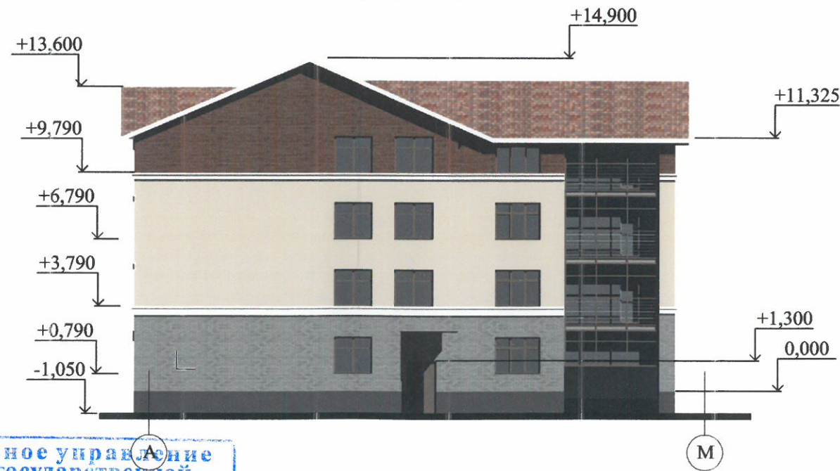
Фасад в осях А - М
